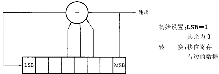
图 11 扰码发生器
