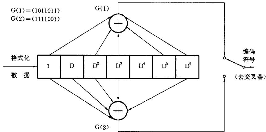
图 9 编码器框图
