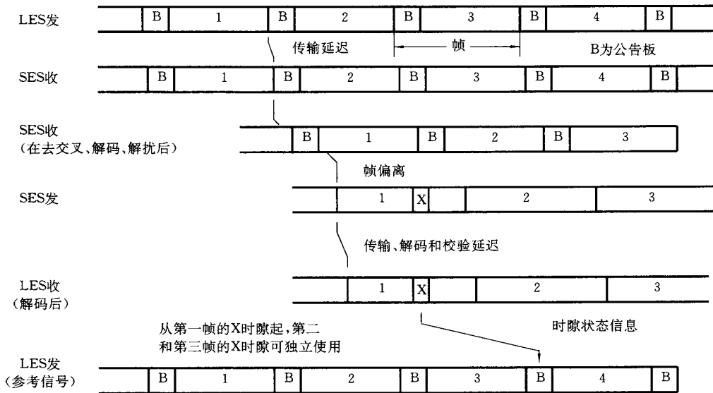
图 14 2 帧时隙的传送过程
