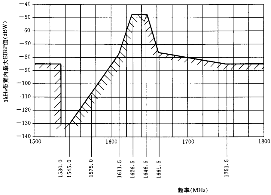
图 5 寄生噪声输出频谱
